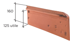
Rive individuelle à emboîtement PV 13 Huguenot (2,7 par ml au pureau de 368 mm) Droite Réf. 215.41
