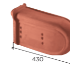
About de rive universelle Gauche Réf. 1070 Droit Réf. 1071
