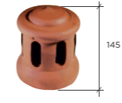
Lanterne modèle Ø 126 (section d'aération 80 cm 2 ) Grand Réf. 1001
