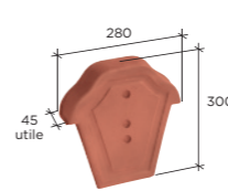
Fronton pour faîtière losangée à recouvrement Réf. 809
