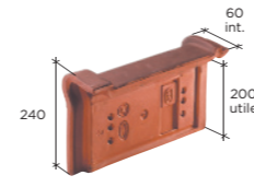
Rive universelle (3 par ml) Réf. 1050
