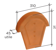
Fronton pour faîtière 1/2 ronde à recouvrement Réf. 807
