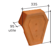
Fronton de rive universelle Réf. 1080
