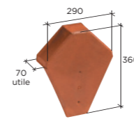
Fronton pour faîtière angulaire à emboîtement Réf. 801
