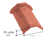
Faîtière losangée à emboîtement (2,5 par ml) Réf. 716
