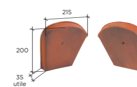
Fronton pour faîtière Shed Droit Réf. 805 Gauche Réf. 806
